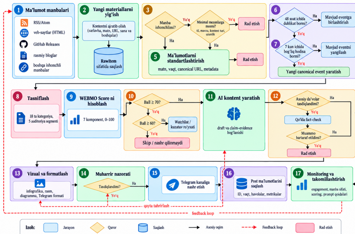
1-rasm. AI yordamida yangiliklarni avtomatik nashr etuvchi botning yakuniy blok-sxemasi
